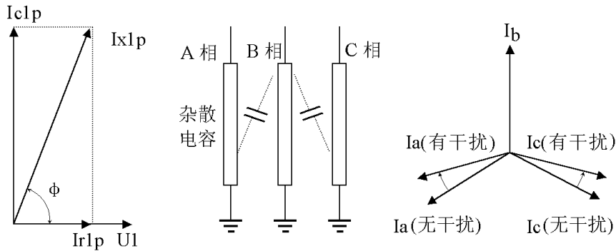
图 8 投影法
