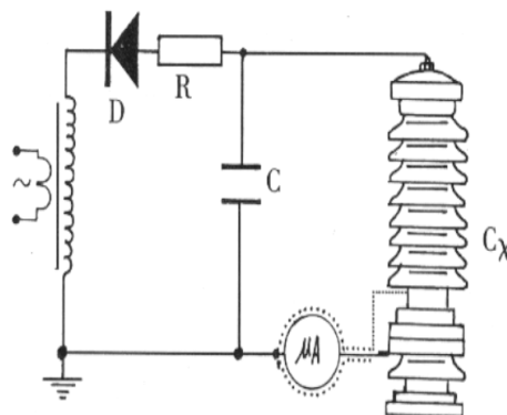
图 7 微安表接入试品 CX 底部的接线图 图 8 排除试品 CX 表面影响接线图
